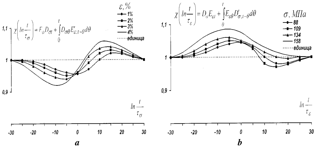
Рисунок 5 - Применение критериев (19) - (а), (20) - (б) с функцией ИВ к текстильной лавсановой нити 114 текс при температуре T = 20^{\circ}C
