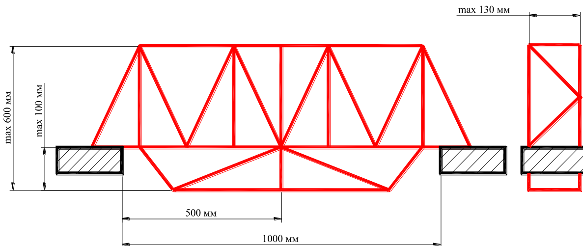
Размеры моста и расположение опор
